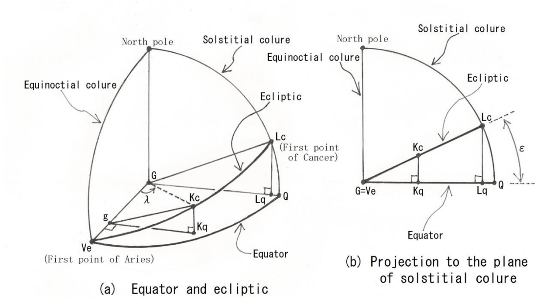
Fig.4, Solar longitude
