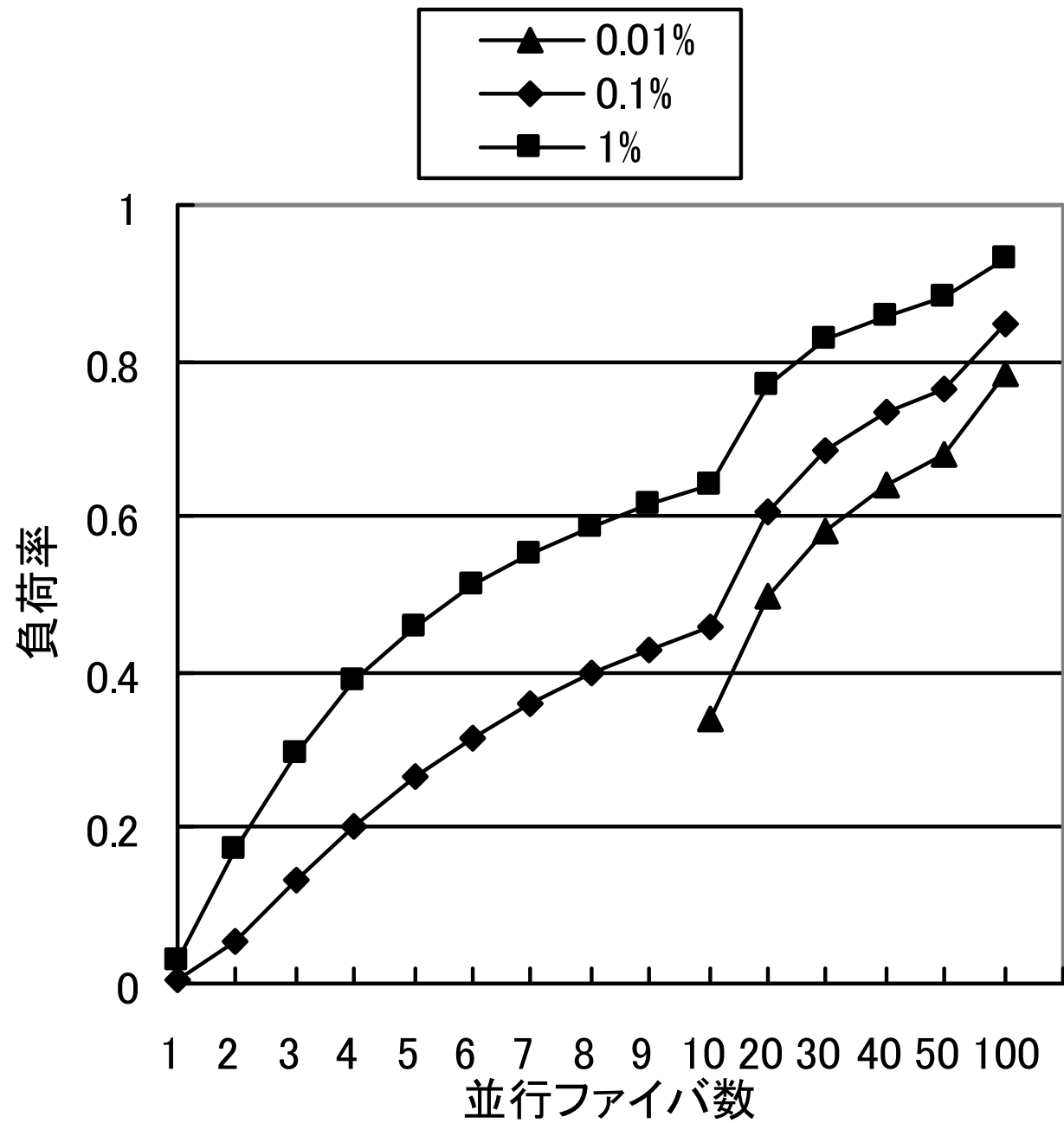
図2 並行ファイバだけの衝突回避
