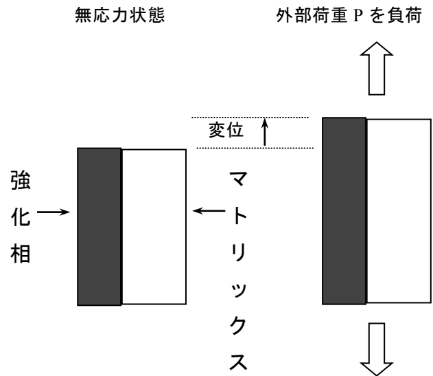
図3 組合せ棒
