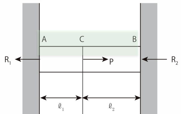
図 2 剛体壁の反力
