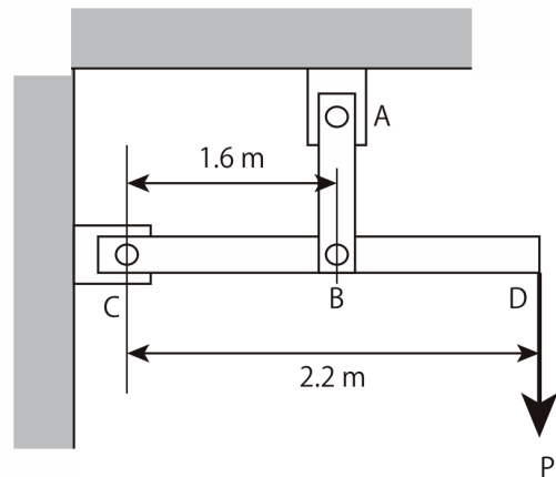
図 1 剛体棒を支える弾性棒
