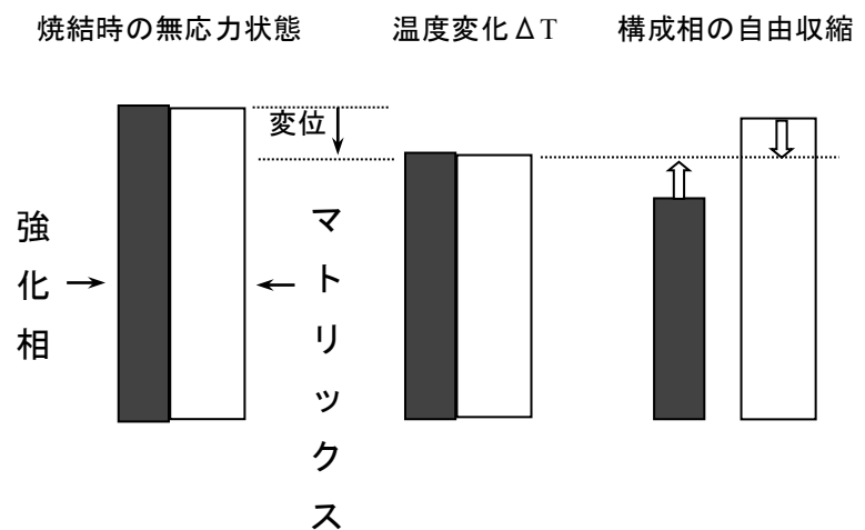
図4 熱応力
