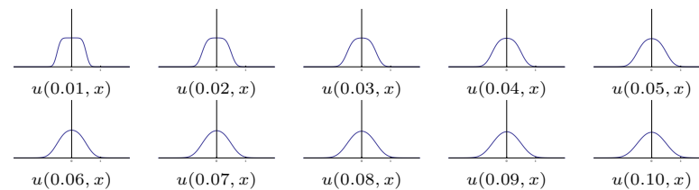
図 8.2 熱方程式の解 (8.13) ( c = 1 )
