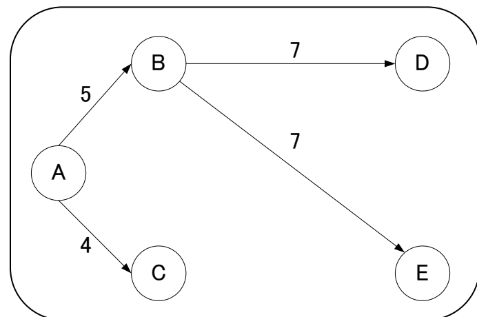
最短路木
