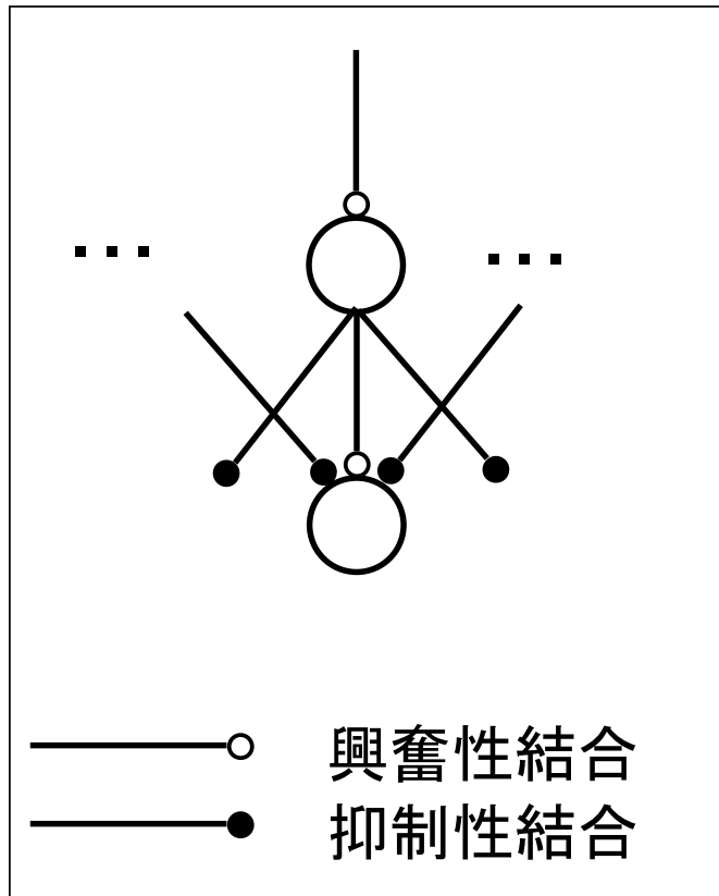
側抑制結合
