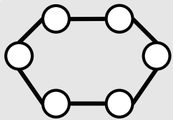
C_6
