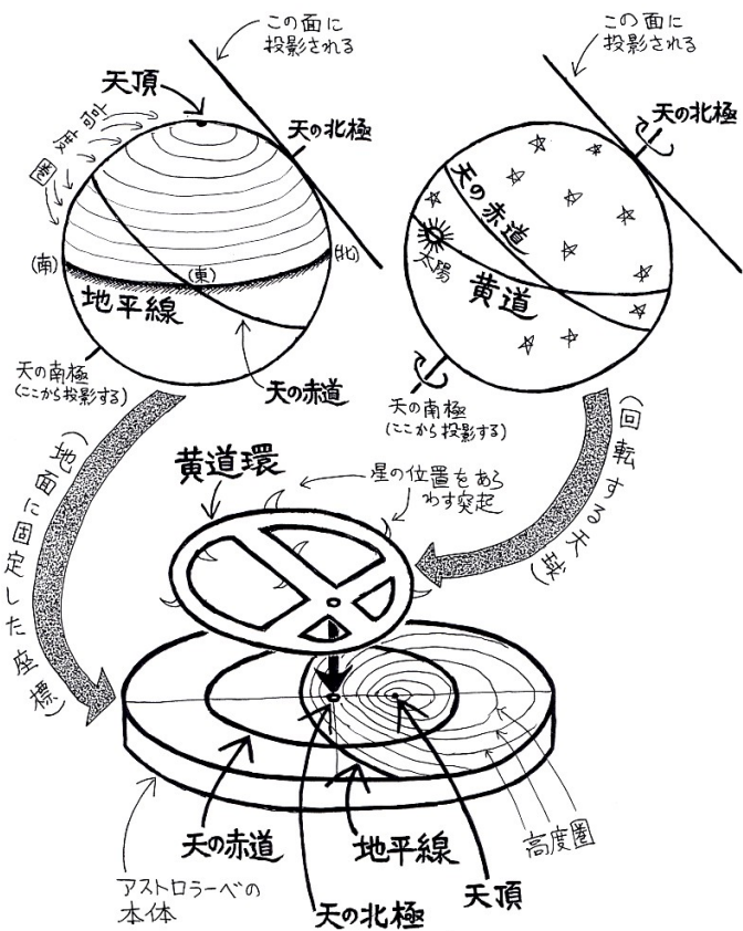
アストロラーベのしくみ (第5図)
