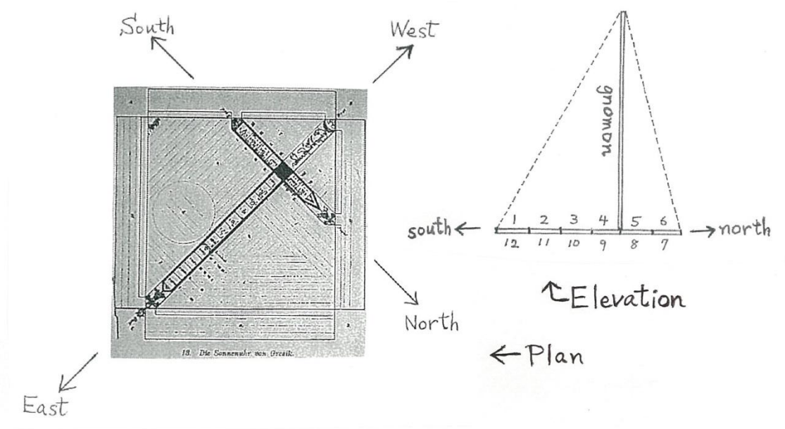
[第 17 図] ジャワのノーモン (Javanese gnomon) (左図の平面図は、Maass (1924, Fig.13) に加筆、右図の立面図は、Maass の記述に基づき筆者作成)
