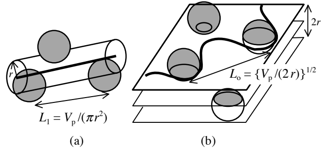
図 11.3 転位線上の平均粒子間隔. (a) 直線転位の場合 ( L_1 ), (b) 完全にフレキシブルに曲がる転位の場合 ( L_o )
