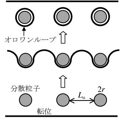
図 11.4 分散強化のオロワン機構
