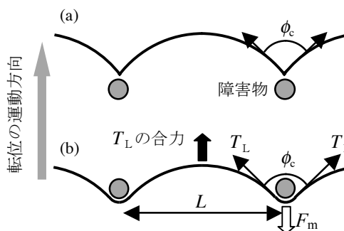
図 11.1 障害物間を張り出す転位。転位と障害物の相互作用は (a) 引力型、(b) 斥力型
