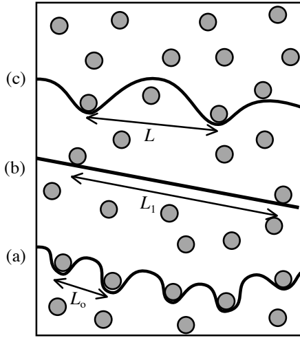
図 11.2 すべり面上の障害物の平均間隔が L_o のとき, (a) 強い障害物, (b) 弱い障害物, (c) 中間的な強さの障害物による転位の曲がり方と転位上の障害物の平均間隔の相異
