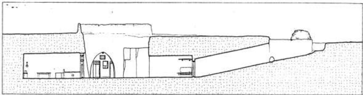
图二 同断面图
