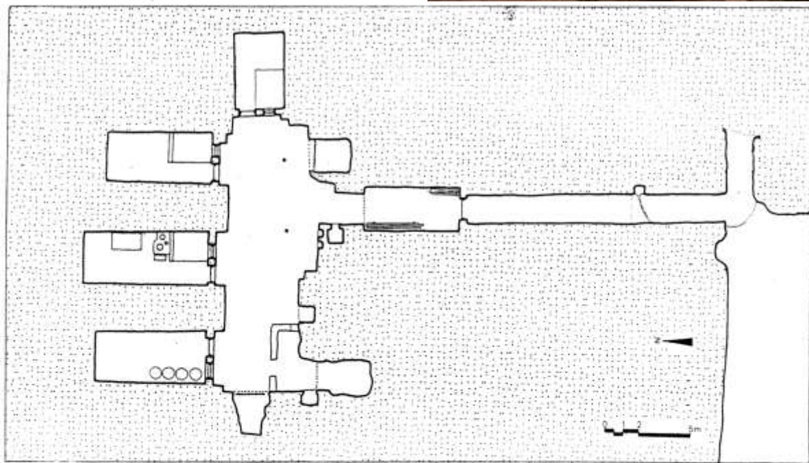
图一 甘肃省庆阳地区华县 秦景厚宅平面图
