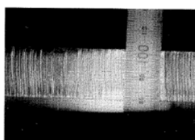
(b) 悪い切断面 (深いドラグライン)
