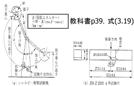
図 3.14 シャルピー衝撃試験
