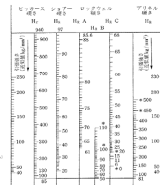
図 3.38 鋼のビッカース硬さに対する近似的換算図表 4) (本図表や*のある範囲内の数値はより高い値を示す)
