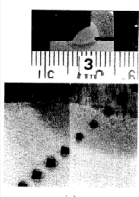
図 3.37 ビッカース硬さ試験によるくぼみと測定例
