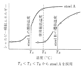
図 3.16 遷移温度アプローチ
