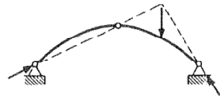
(d) Three hinged arch.
