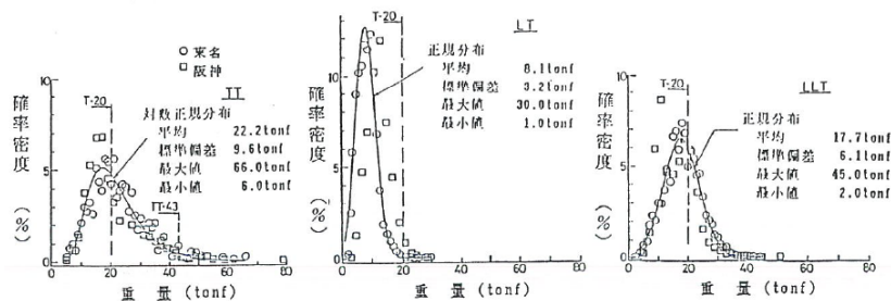
図-3 車両重量分布
