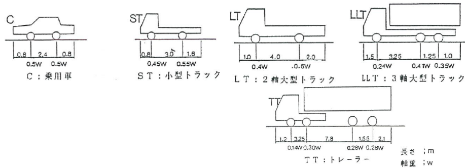
図-2 車両のモデル
