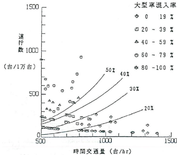
図-8 時間交通量と連行数
