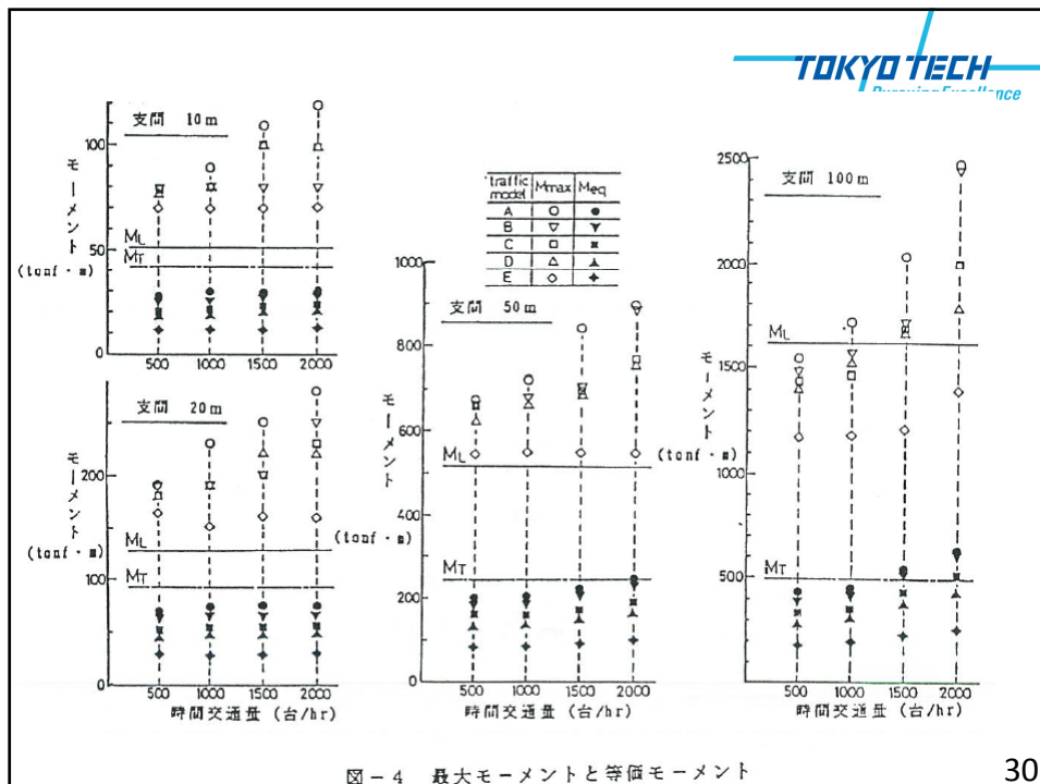
図-4 最大モーメントと等価モーメント
