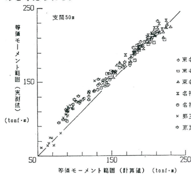
図-9 等価モーメント範囲の実測値と計算値
