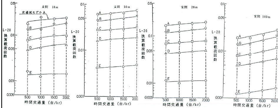
図-11 L-20換算載荷回数
